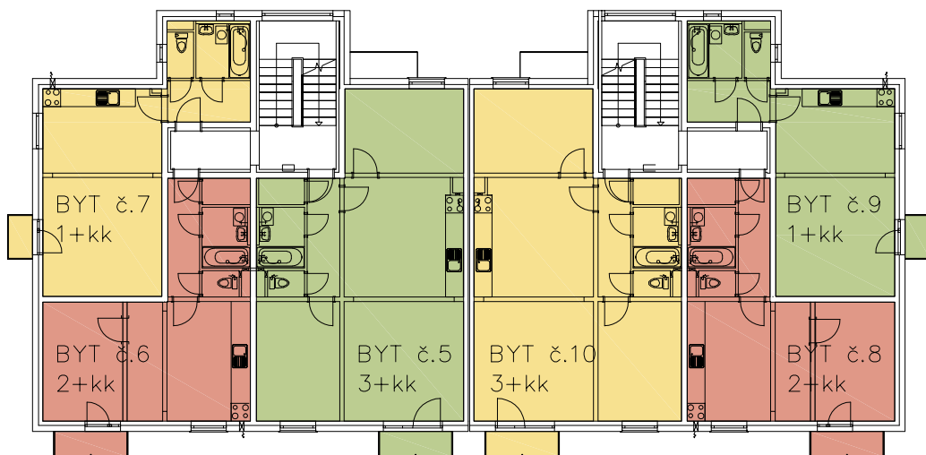
PŪDORYS 2.NP
